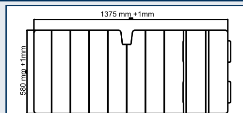
Stanzzeichnung
